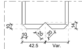
Udskæring til samlings liste
